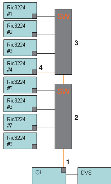
4 sections = 0,5 ms
