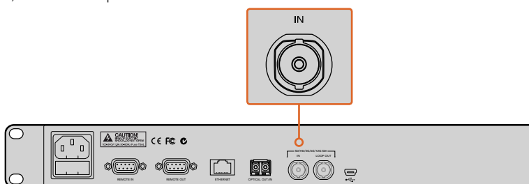
Schließen Sie Ihre Videoquelle an den SDI-Anschluss an. Der Ton ist in das SDI-Signal eingebettet
