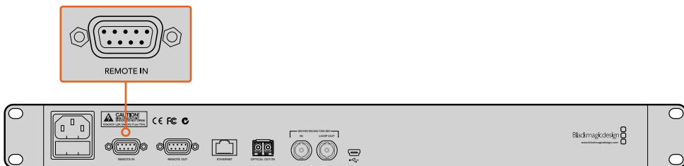
외부 RS-422 컨트롤러를 Blackmagic Duplicator 4K 리모트 입력에 연결하여 기기를 원격으로 제어합니다.
