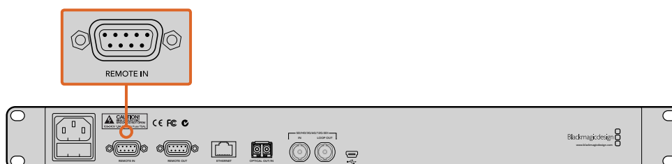
Connetti un dispositivo RS-422 di controllo esterno all'ingresso REMOTE IN di Blackmagic Duplicator 4K per gestire l'unità a distanza.
